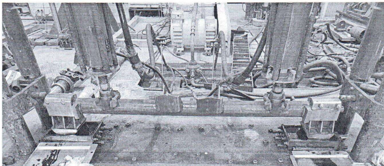
Рисунок 1 – Общий вид балки оси AXL на стенде.
